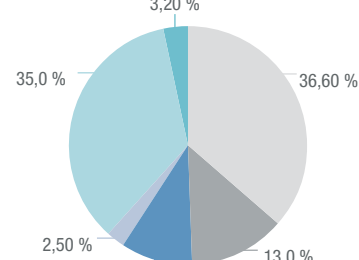
Energieträgermix Deutschland:
